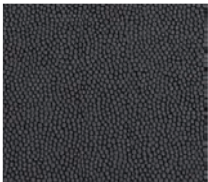
ANTHRACITE SOFTMAX
